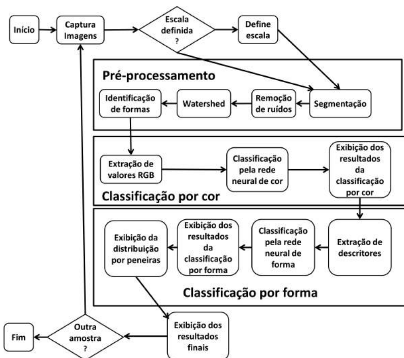
Figura 6. Diagrama de blocos do Qualicafé.
