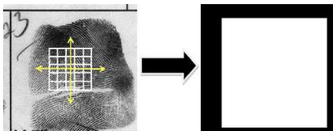
Figura 7. Esquema da obtenção do contorno inicial para uma dada imagem (NIST (2010)). À esquerda, as linhas brancas representam os 25 blocos centrais, os vetores indicam os sentidos da busca e C é a origem dos vetores. À direita, a máscara binária obtida.
