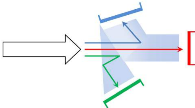
Figura 11. Montagem com 3 sensores para imageamento colorido.
