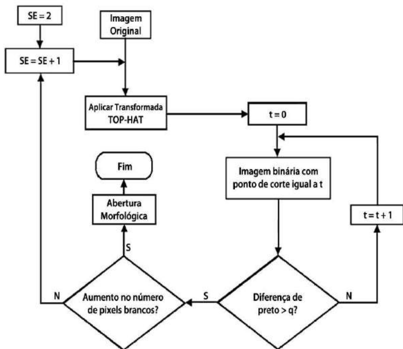
Figura 6. Algoritmo de deteção de manchas.
