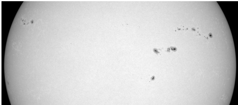
Figura 2. Imagem original com manchas, SOHO.
