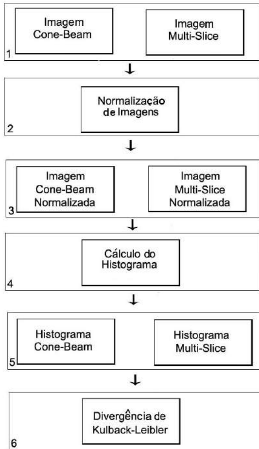
Figura 3. Metodologia proposta.
