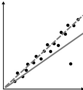
Figura 8. Representação simples de um outlier: o ponto fora da curva
