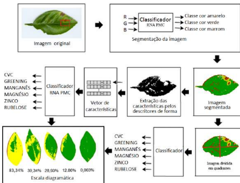
Figura 8. Etapas de processamento: aquisição, segmentação por cor, divisão por quadrante, processamento das doenças, extração de atributos e classificação das doenças com as informações extraídas do vetor de características e geração da escala diagramática.
