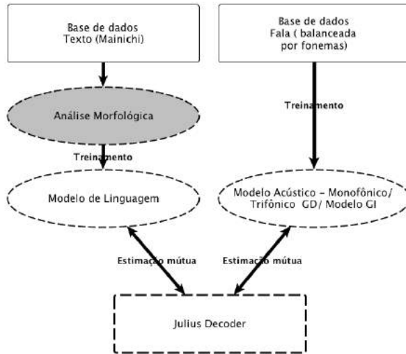
Figura 3. Plataforma LVCSR.
